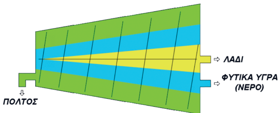
Σχήμα 3. Εκτός του φυγοκεντρωτή δυο φάσεων που είναι ο πιο συνηθισμένος στα ελληνικά ελαιοτριβεία υπάρχουν και αυτοί των τριών και δυο και μισό φάσεων. Στο σχήμα φαίνεται το εσωτερικό ενός φυγοκεντρωτή τριών φάσεων.
